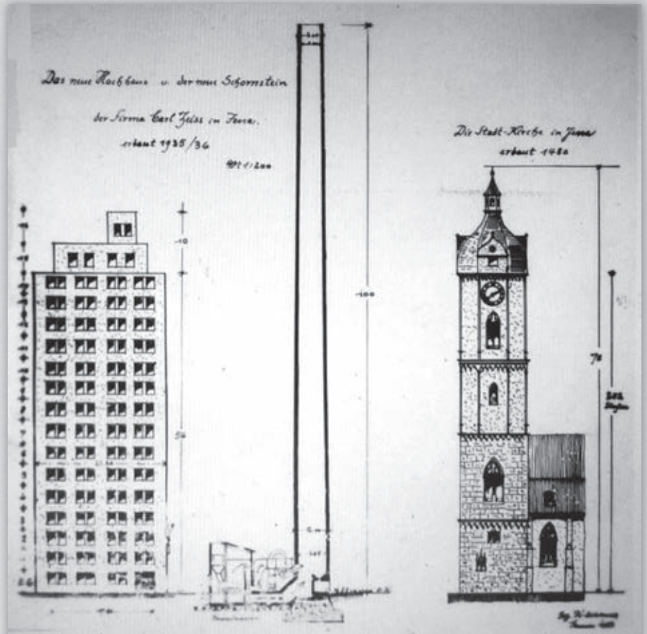
EINE ALTE GRAFIK AUS DEM ZEISS-ARCHIV verdeutlicht die damaligen Größenverhältnisse zwischen dem Ernst-Abbe-Hochhaus am Carl-Zeiss-Platz, dem neuen Schornstein und dem Turm der Stadtkirche
